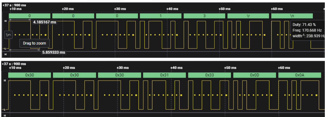
图10. 波形图
