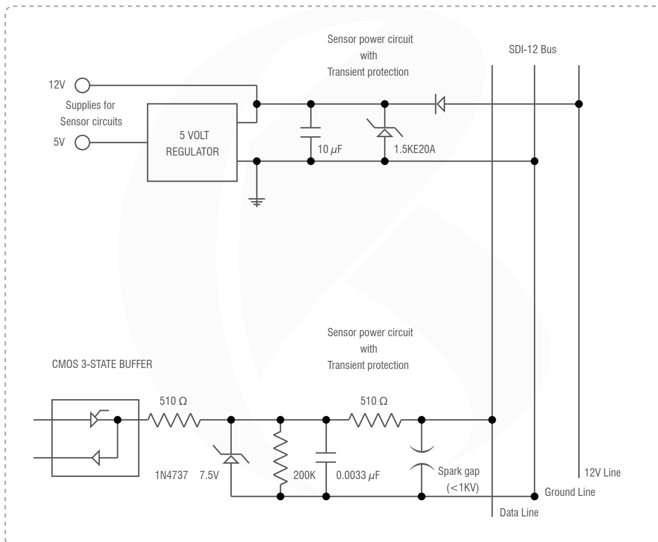
图15. SDI-12推荐电路
