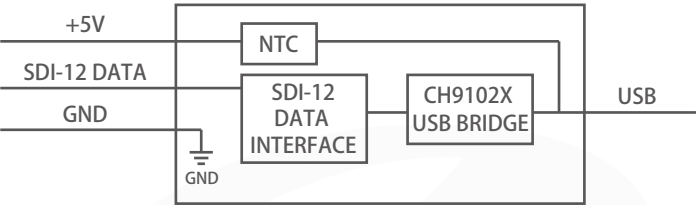
图1. TRS-1201 框图
