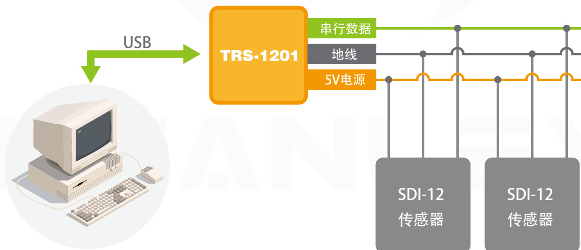
图2. 原理示意
